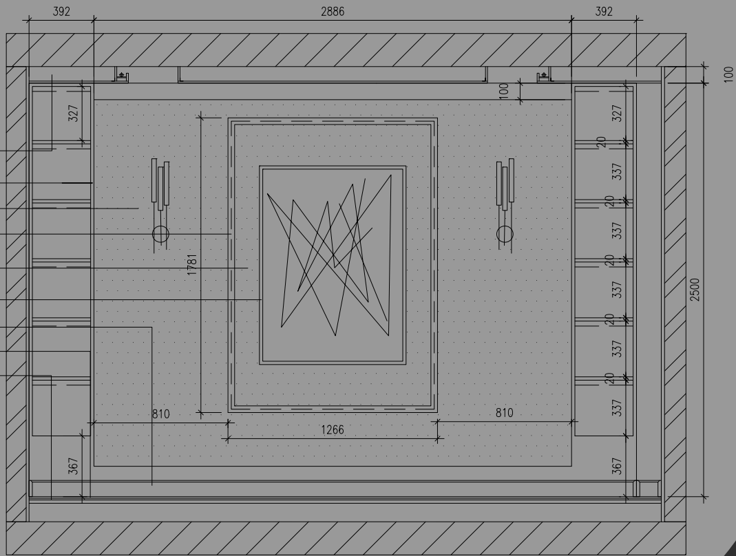
SECTION A-A
